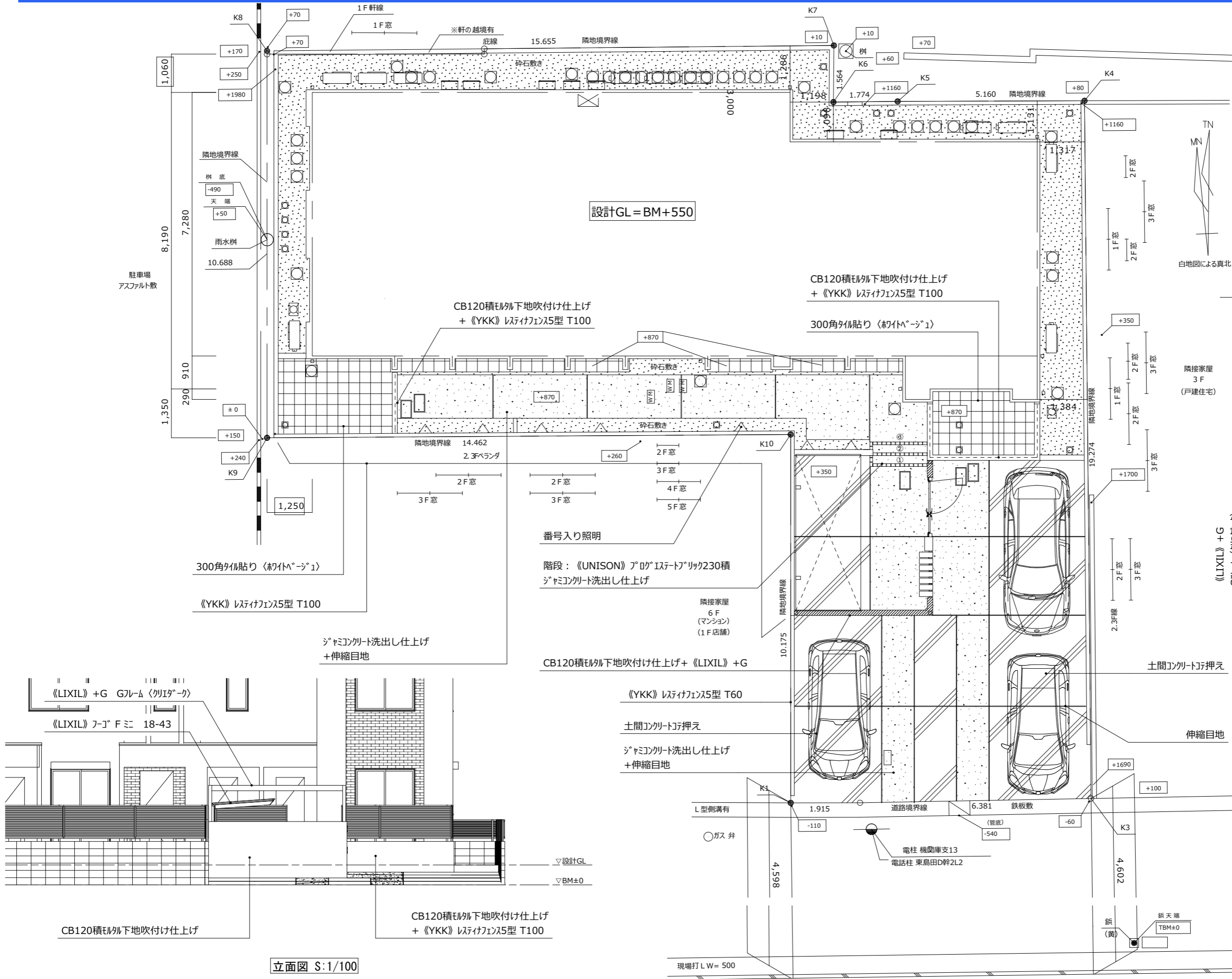
平面図 S:1/100
